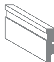
M-01 Altura: 70/100/120/ 150/200mm
